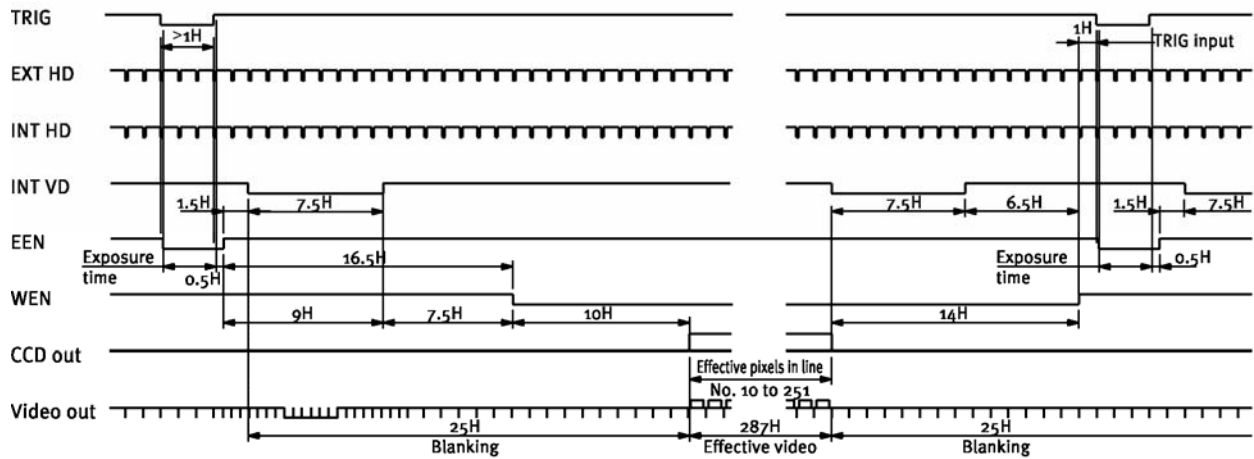
Fig. 19. Pulse width control CCIR.
