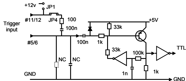
Fig. 5. Trigger input.
