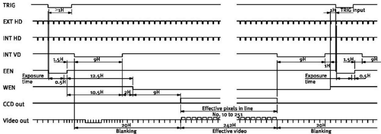
Fig. 18. Edge pre-select EIA
