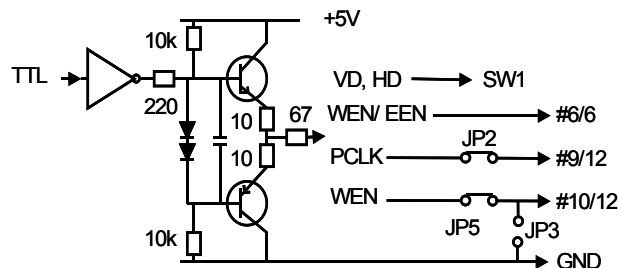
Fig. 7. HD, VD, PCLK, WEN and EEN output.
