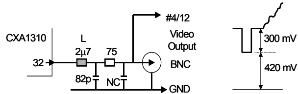
Fig. 4. Video output.
