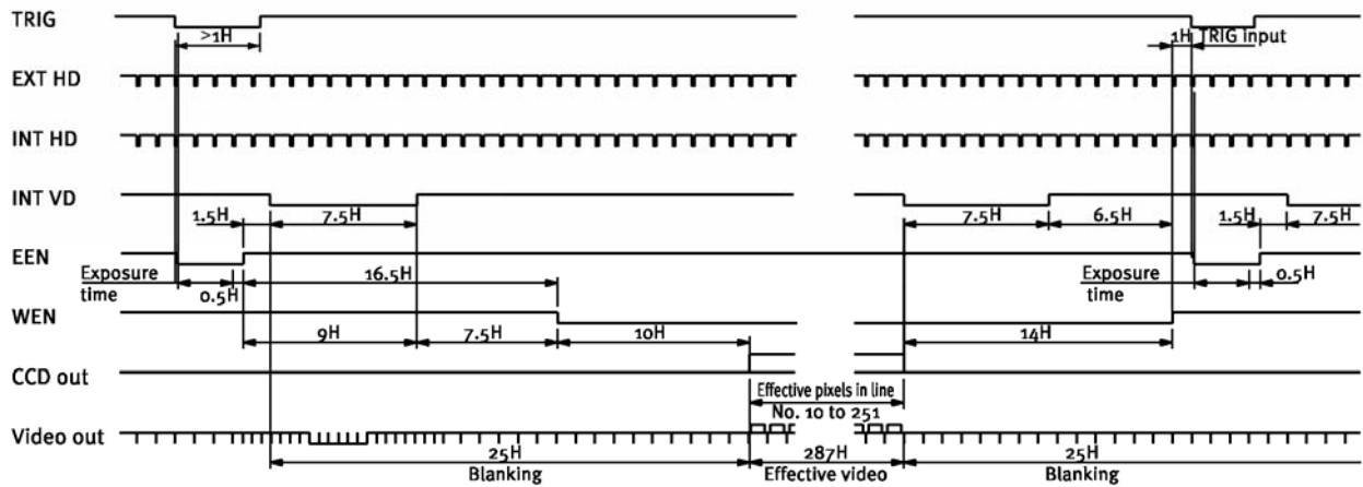
Fig. 17. Edge pre-select CCIR
