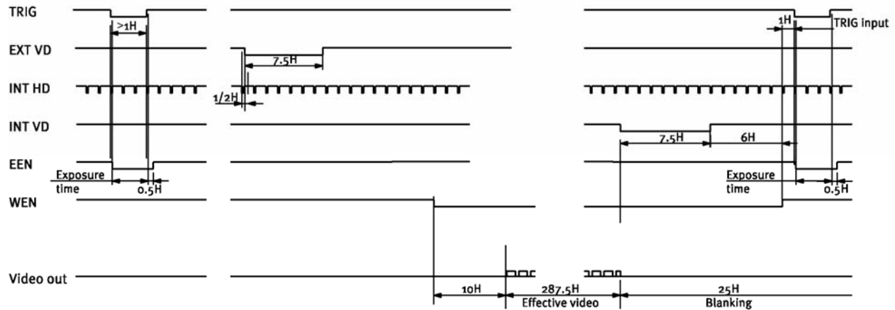
Fig. 21. Frame delay read-out. CCIR
